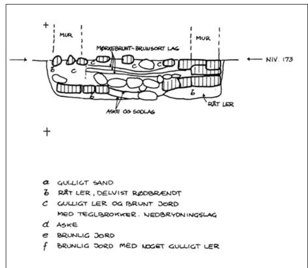
Profiltegning af ovnen – i snittet mellem pilene på oversigtstegningen. Nederst: Ovnens bund
